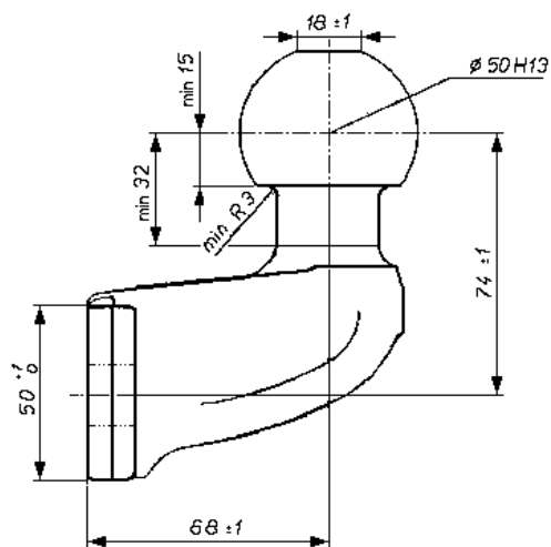
Version 3t und 3,5t
